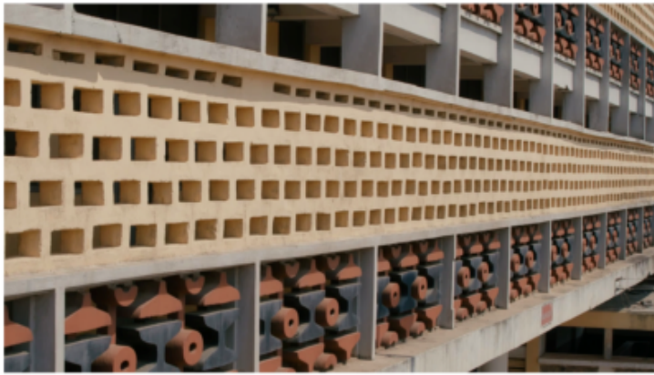
Εικόνα 6: Παραδείγματα κλωστρά από κτήρια που σχεδίασαν οι Fry & Drew στη Γκάνα. Πηγή: film still from Inside mid-century Tropical Modernist architecture | V&A, YouTube28
