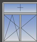
Δίφυλλο ανοιγόμενο - ανακλινόμενο με σταθερό επάνω
